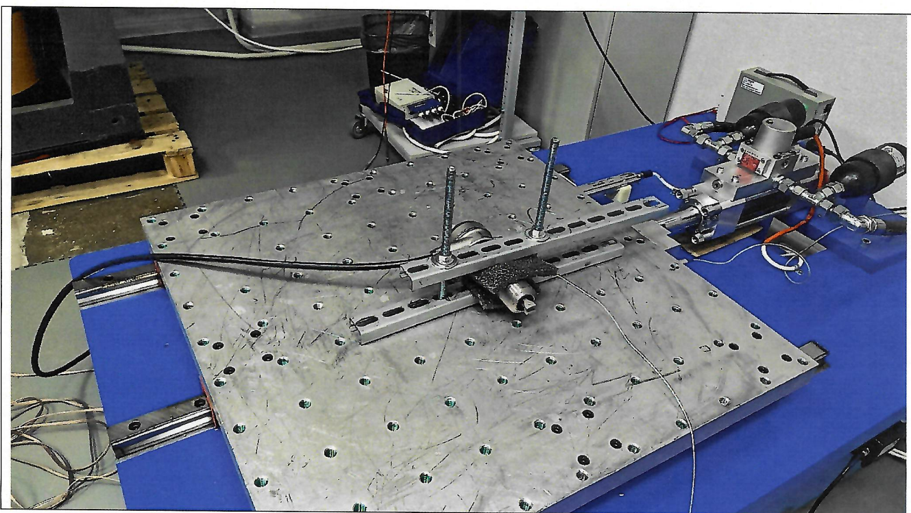
Рисунок 2 Общий вид изделия, закрепленного на платформе вибростенда. При воздействии горизонтально, параллельно каналов кабелей изделия (ось OY).
