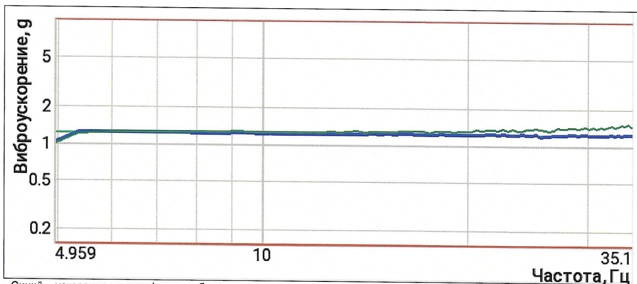
Рисунок А3 – Испытание ПЗ. Направление воздействия, вертикальное по оси OZ.
